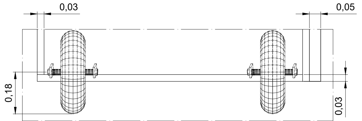
02 DETALHAMENTO ESCALA 1:10
