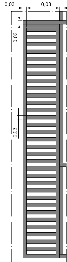
02 DETALHAMENTO 01 ESCALA 1:15
