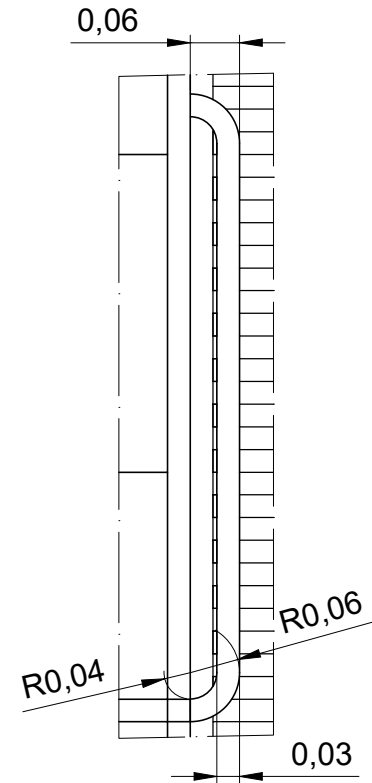
03 DETALHAMENTO 02 ESCALA 1:10
