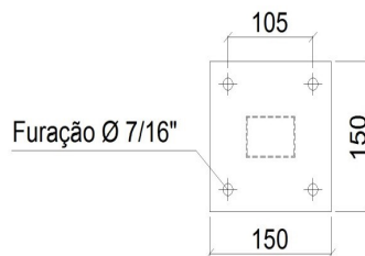
Desenho da base - Vista Superior
