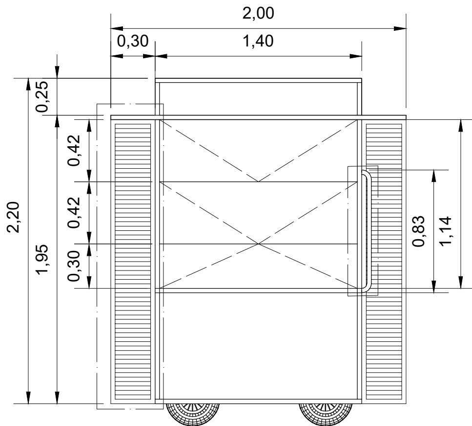
01 VISTA FRONTAL ESCALA 1:25
