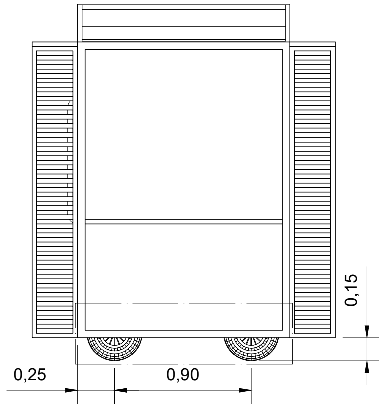
01 VISTA FRONTAL ESCALA 1:25
