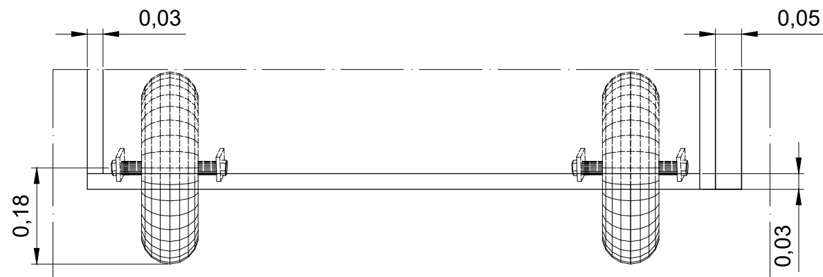
02 DETALHAMENTO ESCALA 1:10
