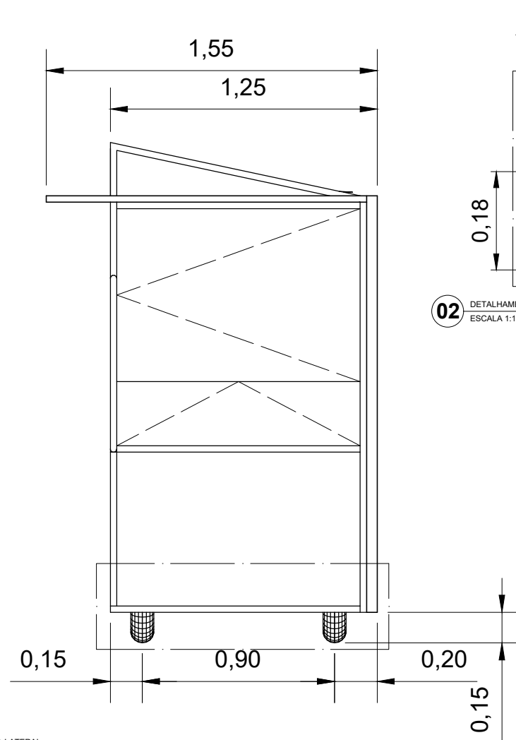
01 VISTA LATERAL ESCALA 1:25
