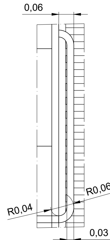
03 DETALHAMENTO 02 ESCALA 1:10
