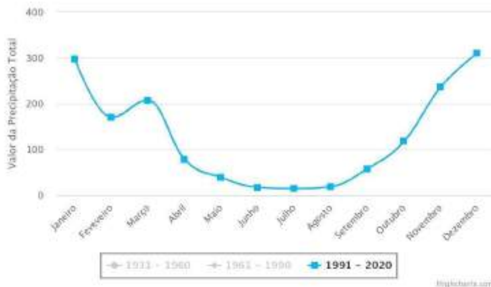
Figura 4 - Precipitação Acumulada (mm) em Juiz de Fora entre os anos de 1991 a 2020
